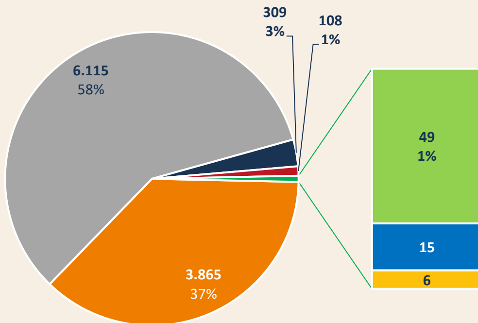
Capacità connessa per classe di potenza del SdA (MWh)
