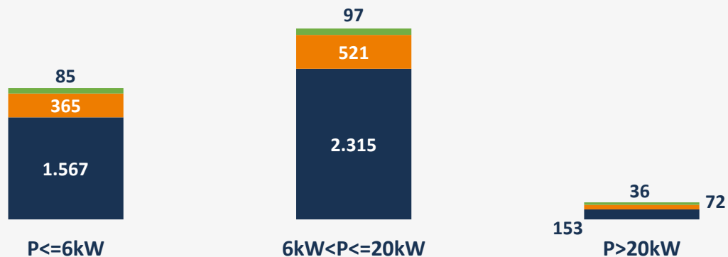
Potenza connessa per tipologia installazione SdA, per classe di potenza del SdA (MW)
